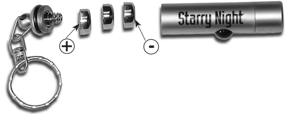
Abbildung 1. Der Pluspol (+) aller drei Batterien muss in Richtung des Schlüsselanhängers (bzw. der Rückseite) weisen und der Minuspol (-) in Richtung der LED (bzw. der Vorderseite) der Taschenlampe.
