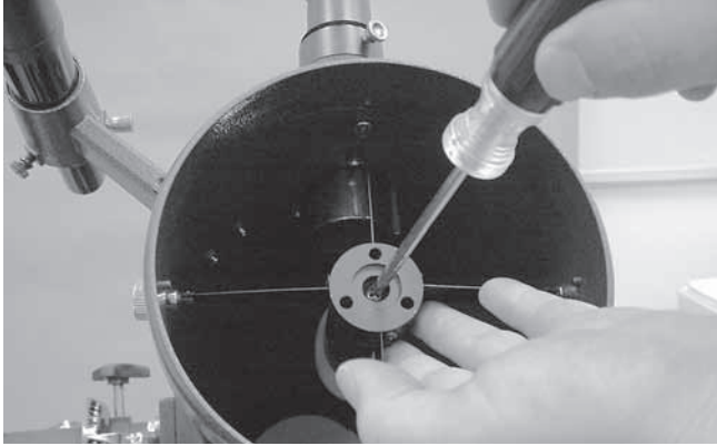
Figura 9. Para centrar el espejo secundario bajo el enfocador, sostenga el soporte del espejo en su lugar con una mano mientras ajusta el tornillo central con un destornillador de estrella. No toque la superficie del espejo
