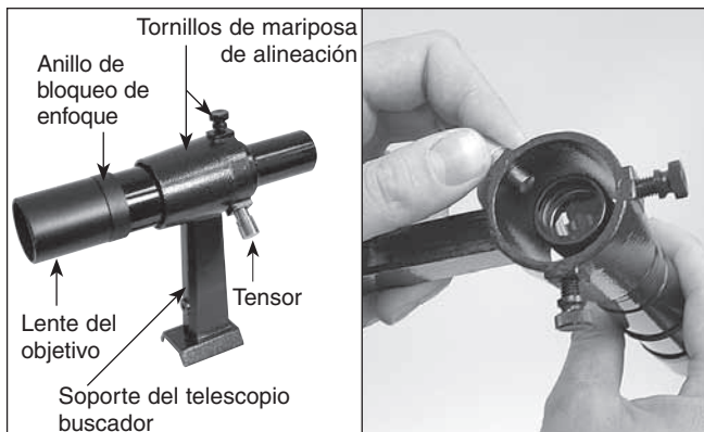
Figura 3a. Telescopio buscador de 6x30.
