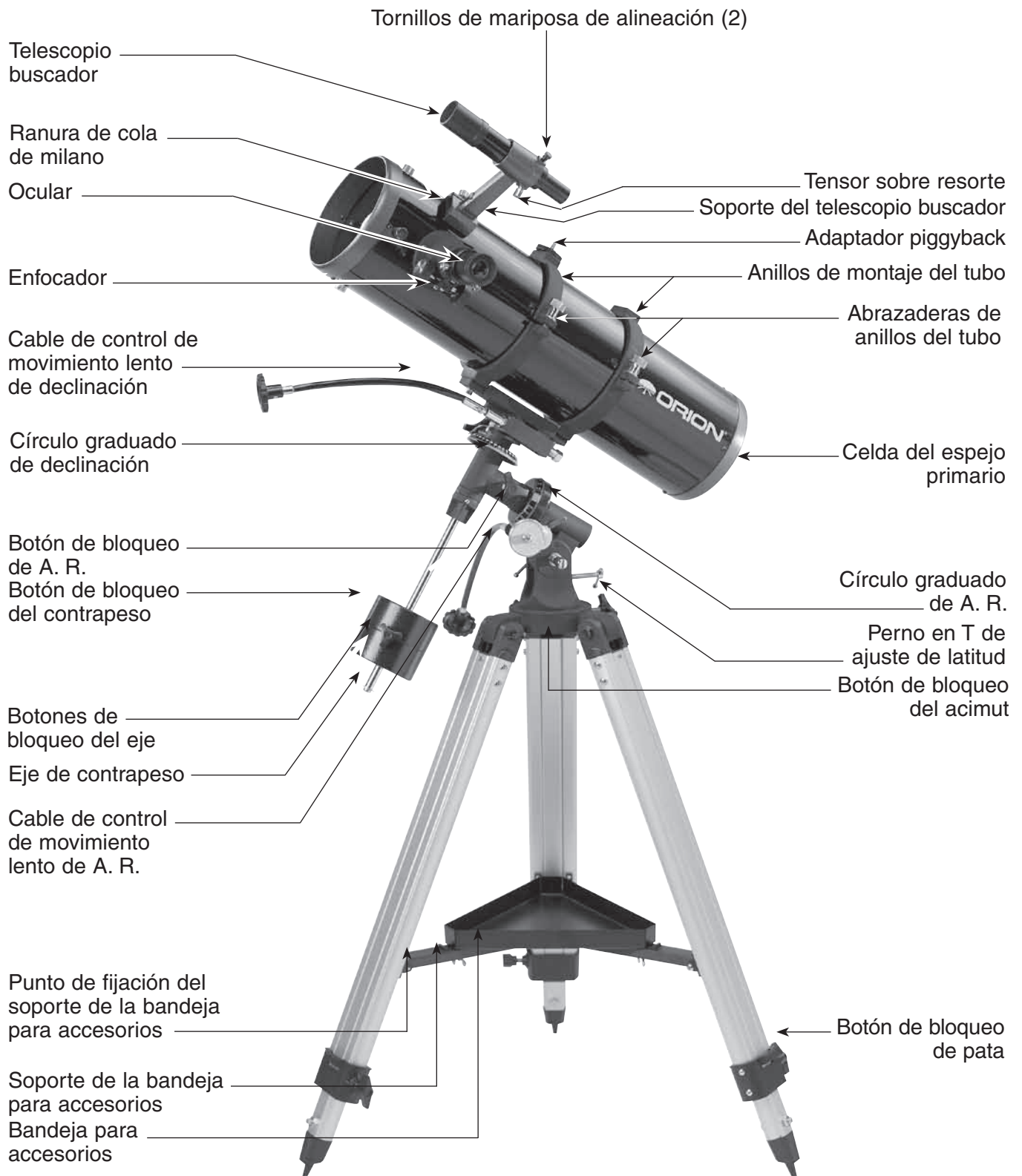
Figura 1. Diagrama de piezas del SpaceProbe 130ST
