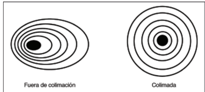
Figura 12. Una prueba de estrella determinará si la óptica de un telescopio está correctamente colimada. Una visión desenfocada de una estrella brillante a través del ocular debería aparecer como se muestra a la derecha si la óptica está perfectamente colimada. Si el círculo es asimétrico, como en la ilustración de la izquierda, el telescopio necesita colimación.
