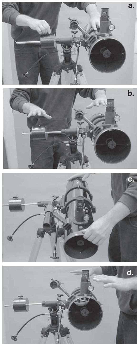
Figura 4. Para un funcionamiento correcto de la montura ecuatorial, es necesario que el tubo del telescopio esté equilibrado en los ejes de ascensión recta y de declinación. (a) Con el botón de bloqueo de A. R. suelto, deslice el contrapeso a lo largo del eje de contrapeso hasta que equilibre exactamente el tubo. (b) Al retirar las manos, el tubo no debe subir ni bajar. (c) Con el botón de bloqueo de Dec. suelto, afloje las abrazaderas de bloqueo de los anillos del tubo un par de vueltas y deslice el telescopio hacia adelante o hacia atrás por los anillos del tubo. (d) Cuando el tubo se equilibra respecto al eje de la declinación, no se moverá cuando lo suelte.
