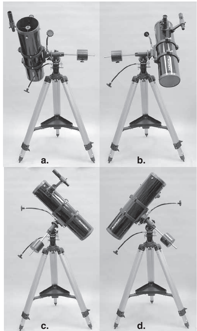
Figura 7. Esta ilustración muestra el telescopio apuntando a los cuatro puntos cardinales (a) norte (b) sur (c) este (d) oeste. Observe que el trípode y la montura no se han movido, solo se ha desplazado el tubo del telescopio en los ejes de ascensión recta y declinación.
