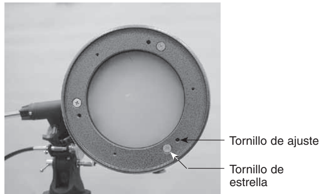
Figura 11. Extremo posterior del tubo óptico (parte inferior de la celda del espejo primario). Los tres pares de tornillos de ajuste y tornillos de estrella ajustan la inclinación del espejo primario.
