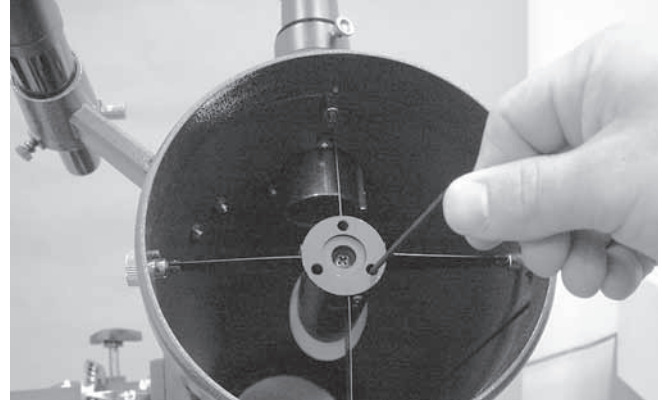
Figura 10. Ajuste la inclinación del espejo secundario, aflojando o apretando los tres tornillos de ajuste de alineación con una llave Allen de 2 mm.
