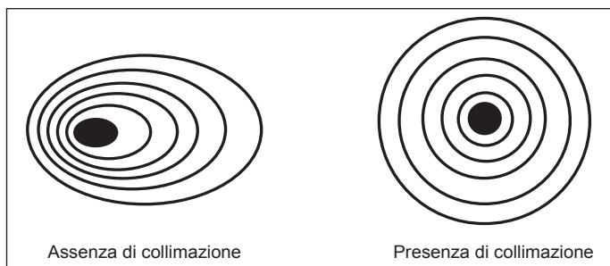
Figura 12. L'osservazione di una stella consente di determinare il grado di collimazione delle ottiche di un telescopio. In presenza di collimazione, l'immagine di una stella luminosa non messa a fuoco attraverso l'oculare dovrebbe apparire come illustrato sulla destra. Se il cerchio non è simmetrico, come nella figura a sinistra, occorre procedere alla collimazione del telescopio.
