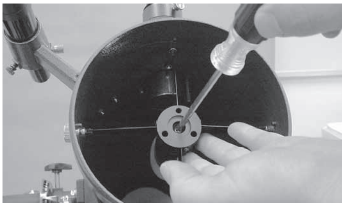
Figura 9. Per centrare lo specchio secondario sotto il focheggiatore, mantenere in posizione il supporto dello specchio secondario con una mano mentre si regola la vite centrale con un cacciavite a croce. Non toccare la superficie dello specchio
