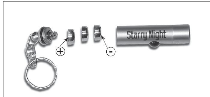
Figure 1. Le pôle positif (+) de l'ensemble des trois piles doit être du côté de la chaînette au bout de la mini-torche et le pôle négatif (-) de la batterie du côté de la LED, à l'avant de la mini-torche.
