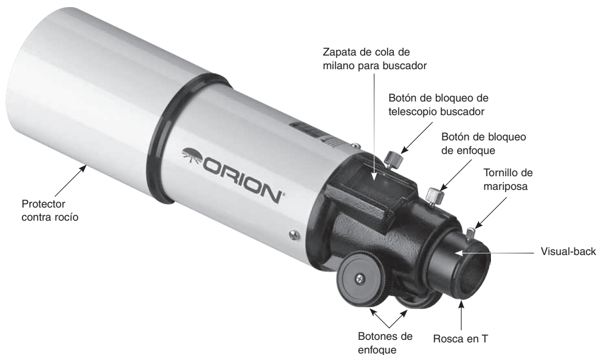
Figura 1. Conjunto de tubo óptico ShortTube 80
